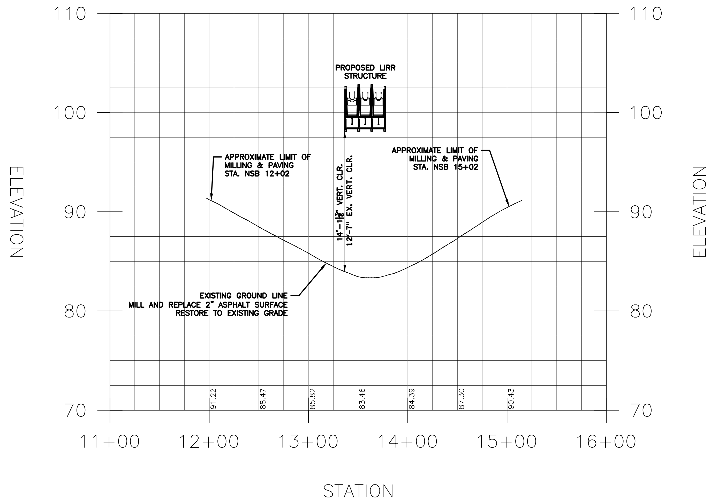
PROFILE – NASSAU BLVD STA. 11+00 TO STA 16+00 HORIZONTAL SCALE: 1" = 50' VERTICAL SCALE: 1" = 5'
